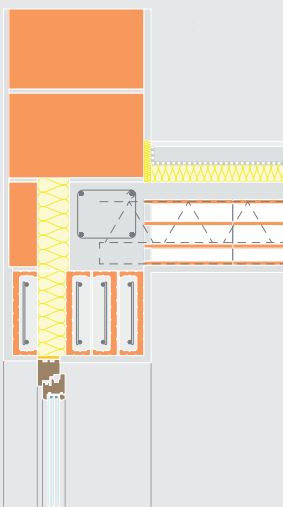
Ściana gr. 38 cm
